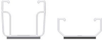
Kortprofil C47 med EPDM 200 mm
