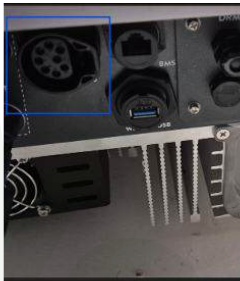
2 Tilslut COM-stikket
